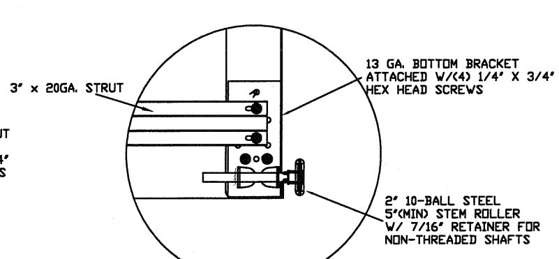
TYPICAL BOTTOM BRACKET N.T.S. ⑤
