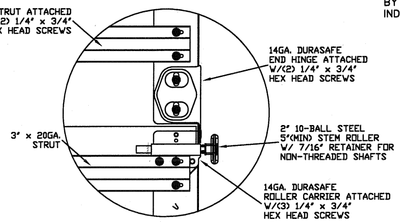
TYPICAL DURASAFE END HINGE N.T.S. ④
