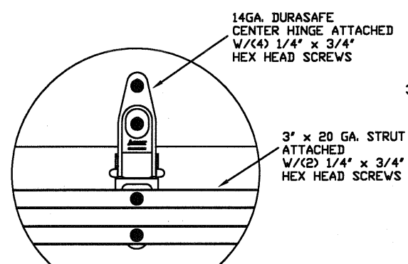
TYPICAL DURASAFE CENTER HINGE N.T.S. ②
